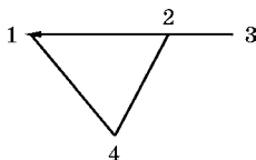
Рис. 28 Существование (1, 3) -маршрута
