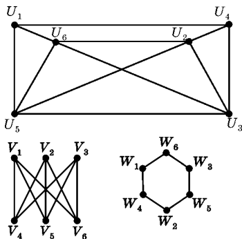
Рис. 9 Изоморфные графы
