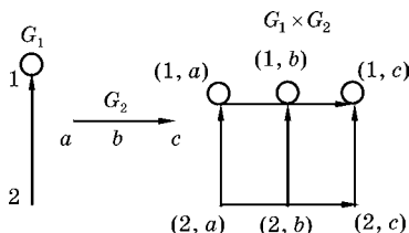
Рис. 20 Произведение графов
