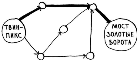
НЕВЗВЕШЕННЫЙ ГРАФ (ПОИСК В ШИРИНУ)
