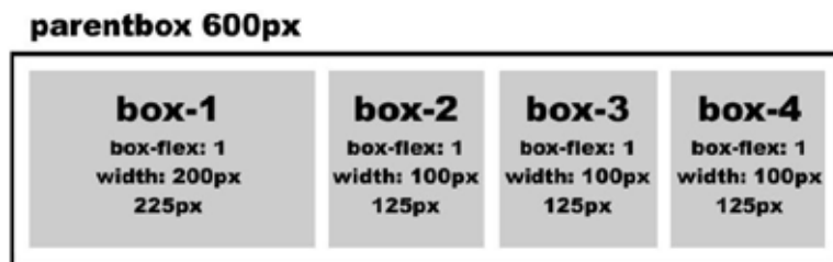
Рис. 2.14. Добавление свободного пространства к значениям ширины всех блоков
